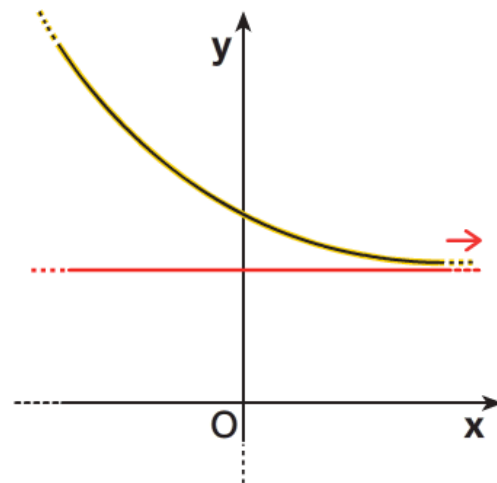
b. Asintoto orizzontale soltanto per x \rightarrow +\infty .
