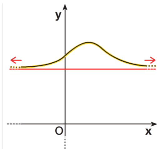
c. Asintoto orizzontale unico per x \rightarrow +\infty e x \rightarrow -\infty .
