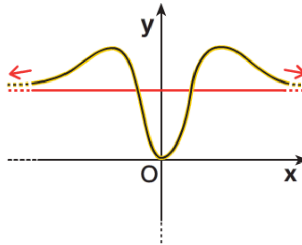
b. Il grafico interseca l'asintoto in due punti.
