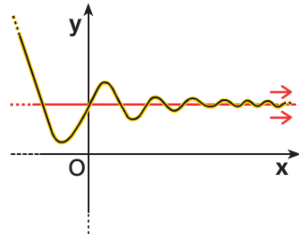
c. Il grafico interseca l'asintoto in infiniti punti.
