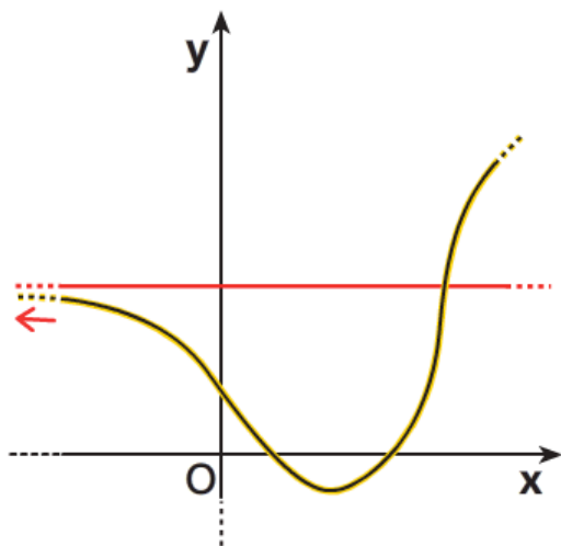
a. Asintoto orizzontale soltanto per x \rightarrow -\infty .
