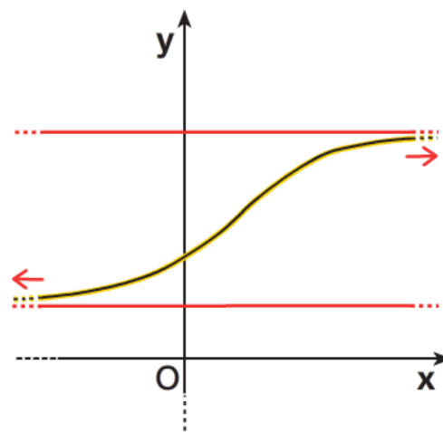
d. Due asintoti orizzontali diversi per x \rightarrow +\infty e x \rightarrow -\infty .
