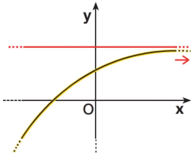
a. Il grafico non interseca l'asintoto.
